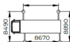
STABILISATEURS (ZONE MAXIMALE DE TRAVAIL)
