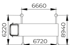
DIMENSIONS DES STABILISATEURS AVEC DÉPLOIEMENT MAXIMAL
