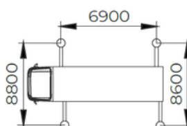
STABILISATEURS (ZONE MAXIMALE DE TRAVAIL)
